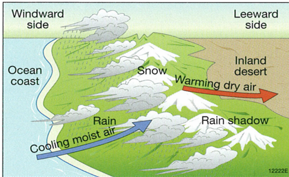
M4 Relief rainfall
